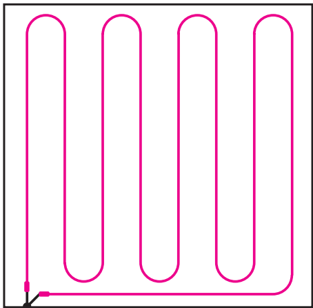
Схема установки одножильного кабеля
